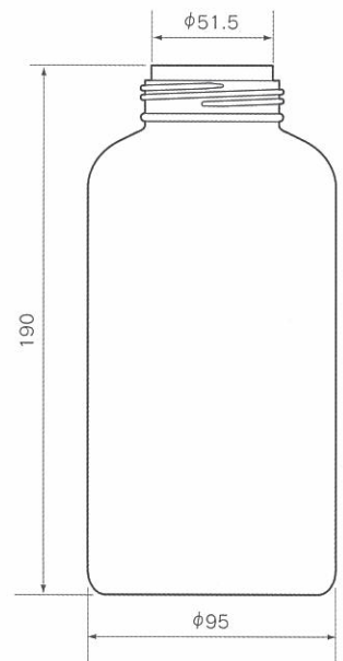
TRI-1000H 広口 入数:50入 OF:1100cc 成形方法:DB 材質:トライタン
