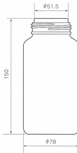
TRI-500H 広口 入数:50入 OF:580cc 成形方法:DB 材質:トライタン
