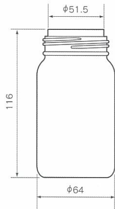
TRI-250H 広口 入数:100入 OF:310cc 成形方法:DB 材質:トライタン
